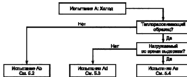
Рисунок 1 — Блок-схема испытаний А: Холод
